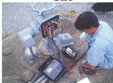
DC4-20mA調整
